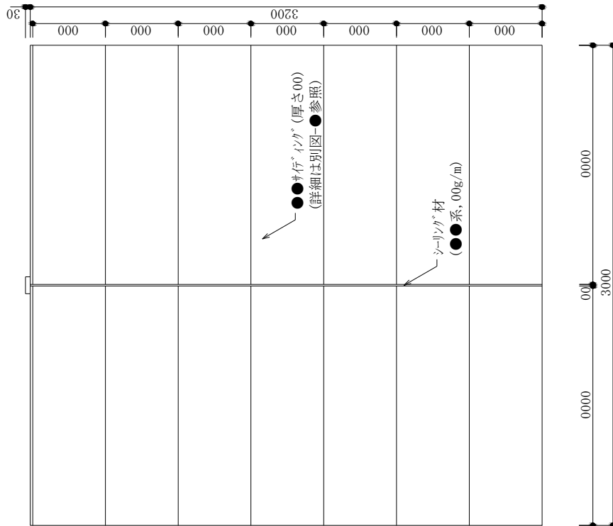
サイディング割付図
