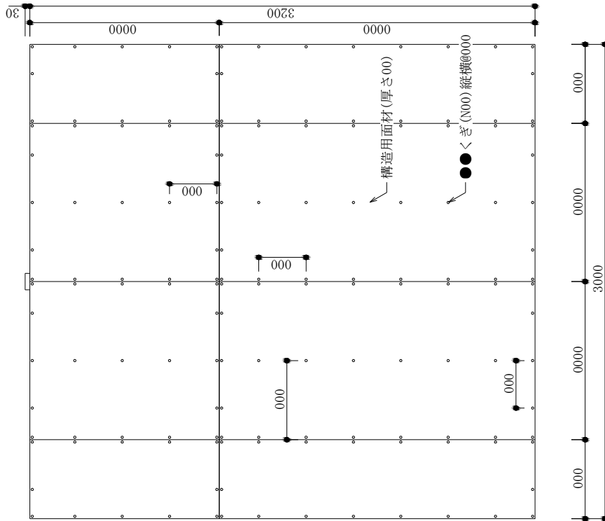
構造用面材割付図
