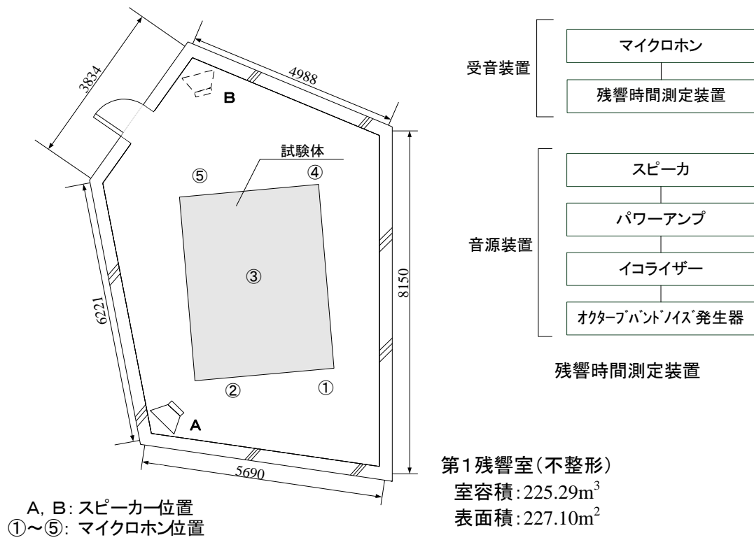
図* 吸音性能試験装置の構成
