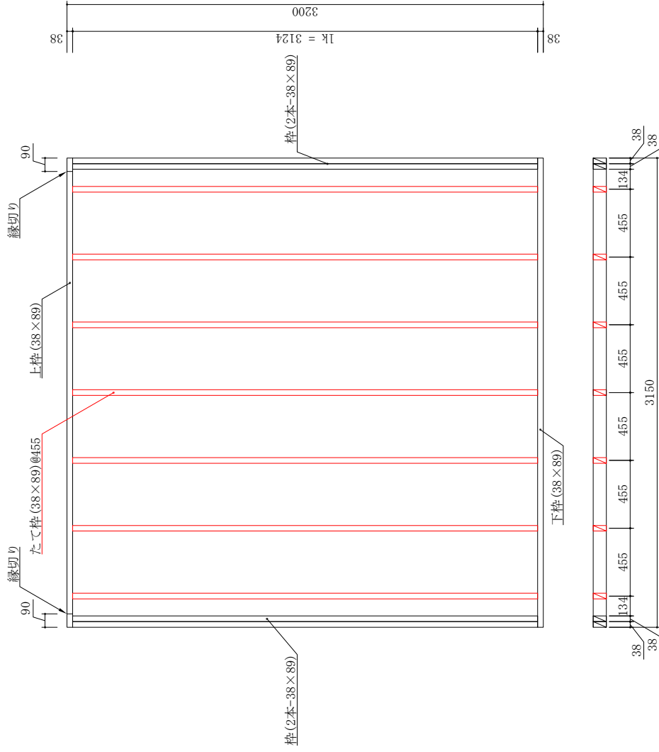
枠組構成図
