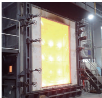
鋼製窓の遮炎性試験
