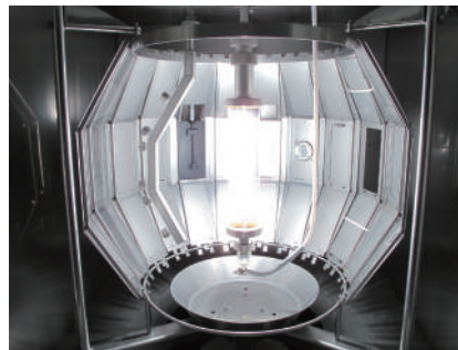
スーパーキセノンウェザーメーター
