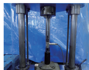
■ 木質構造用ねじのねじり試験
