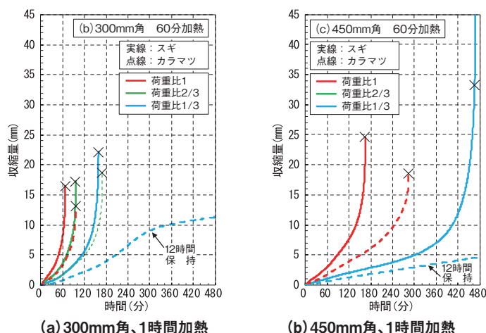
図1 柱の収縮量に関する実験結果 2)
