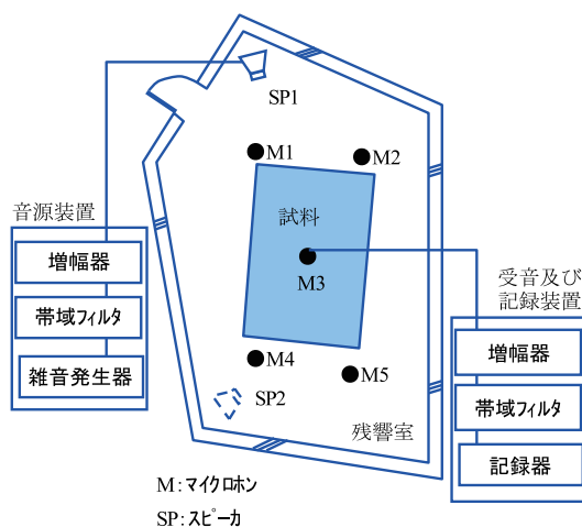
解説図1 試験装置の概要
