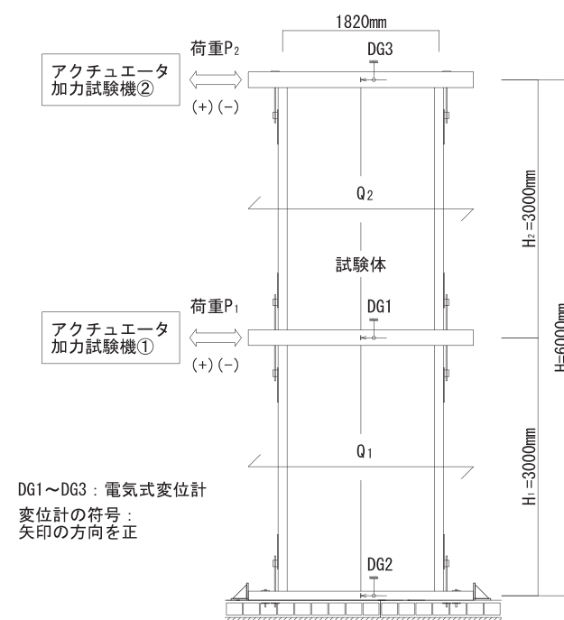
図5 試験方法
