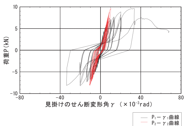
図6 荷重P—見掛けのせん断変形角 \gamma 曲線
