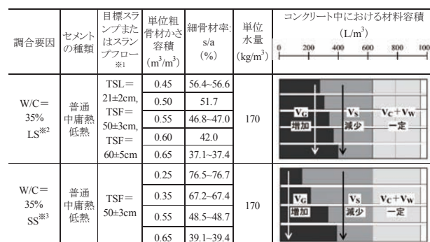
図8 本研究において対象としたコンクリート中の構成割合
