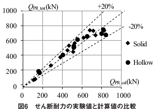
図6 セン断耐力の実験値と計算値の比較
