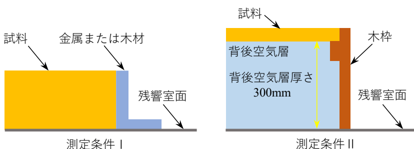
図3 標準測定条件 (JIS A 6301 附属書A)
