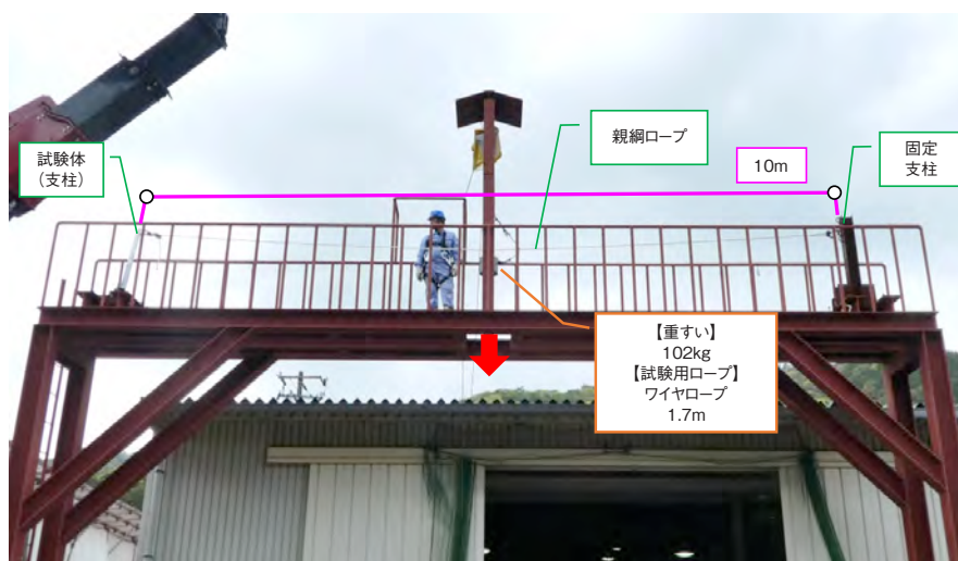
写真1 試験実施状況
