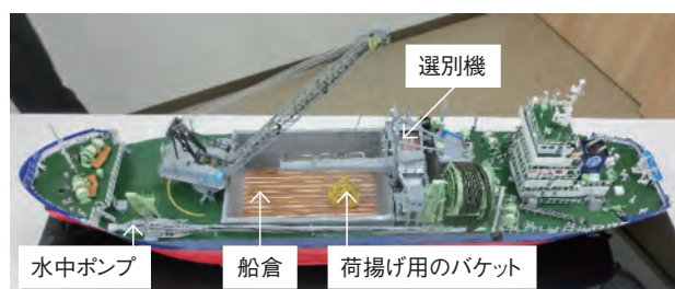
写真3 海砂採取船の模型
