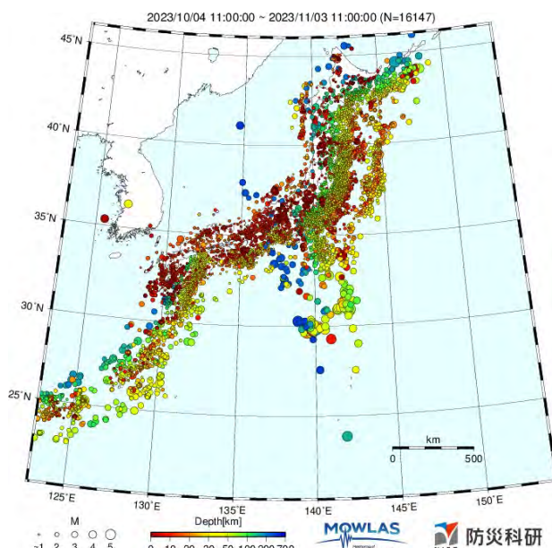
図2 震央分布図
