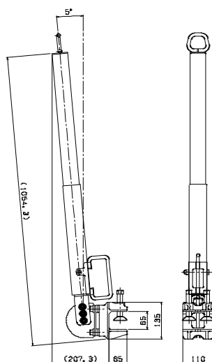
図1 試験体
