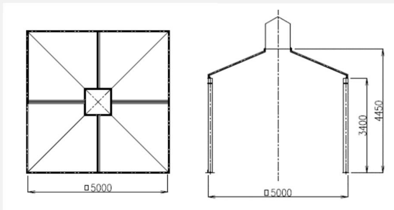
集煙フード
